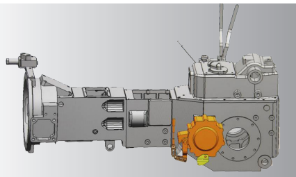
Tugevdatud jõülekanne
