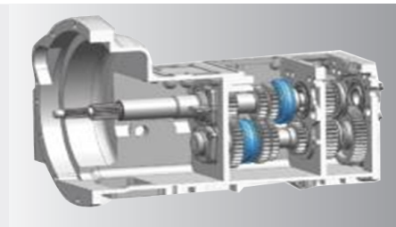
12+12 käiguosa
